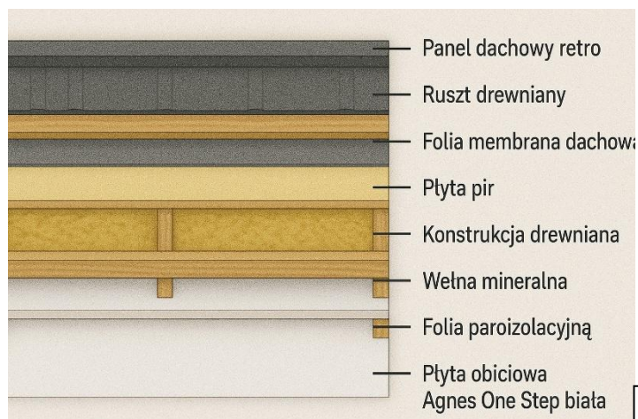
KONSTRUKCJA DACHU
