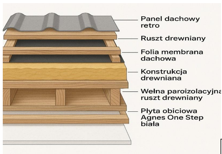
KONSTRUKCJA DACHU
