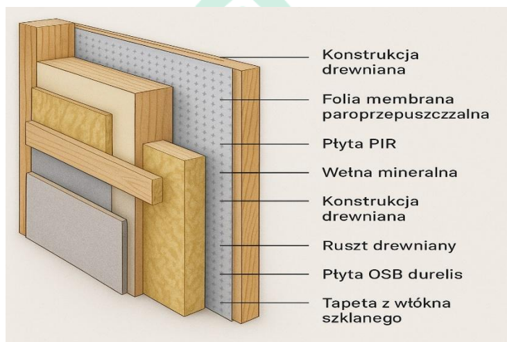
KONSTRUKCJA ŚCIAN
