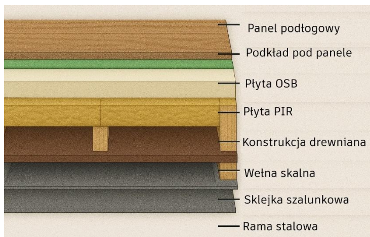
KONSTRUKCJA PODŁOGI
