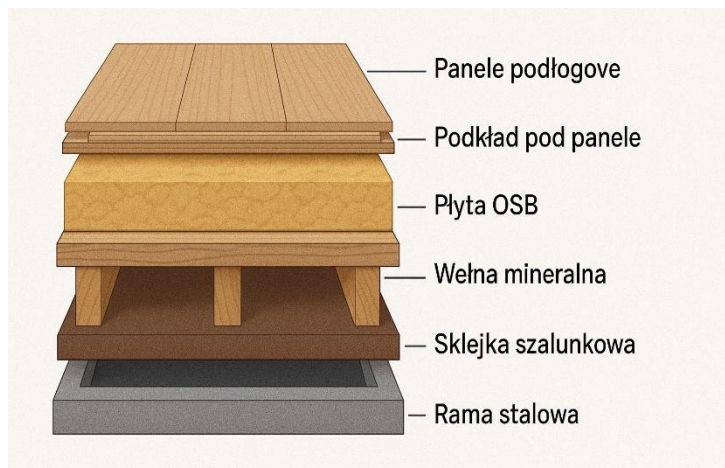
KONSTRUKCJA PODŁOGI
